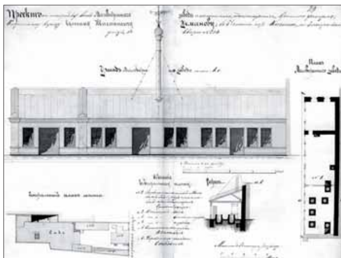
Проект мыловаренного завода Султана Жиганина. Казань. 1898 г.
