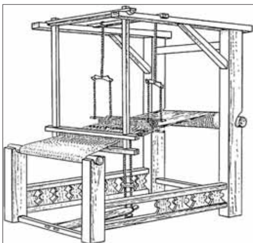
Ручной ткацкий станок. XIX в.
